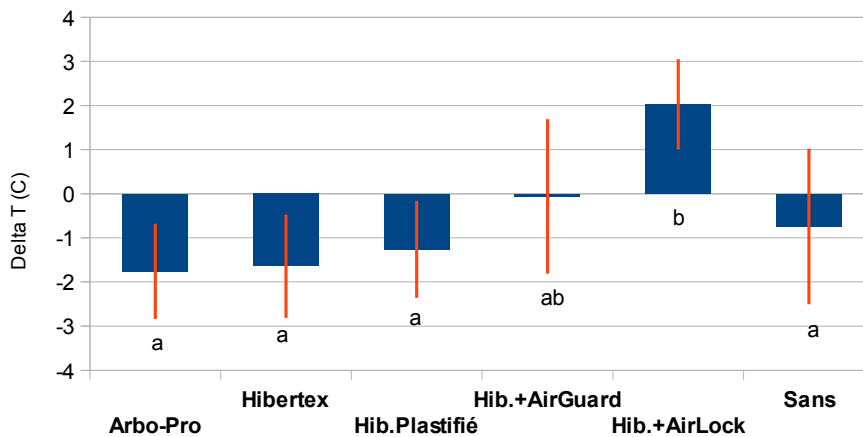
Différence de température à la surface du sol sous les toiles p/r au sol dans l'allée par un après-midi chaud et plutôt nuageux de printemps (T air = 17 °C)
