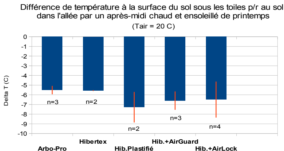
Illustration 14: Différence de température du sol sous les systèmes et celle au centre de l'allée, par un après-midi chaud et ensoleillé de printemps (sans neige, 19 avril 2012). `n` indique le nombre d'observations.
