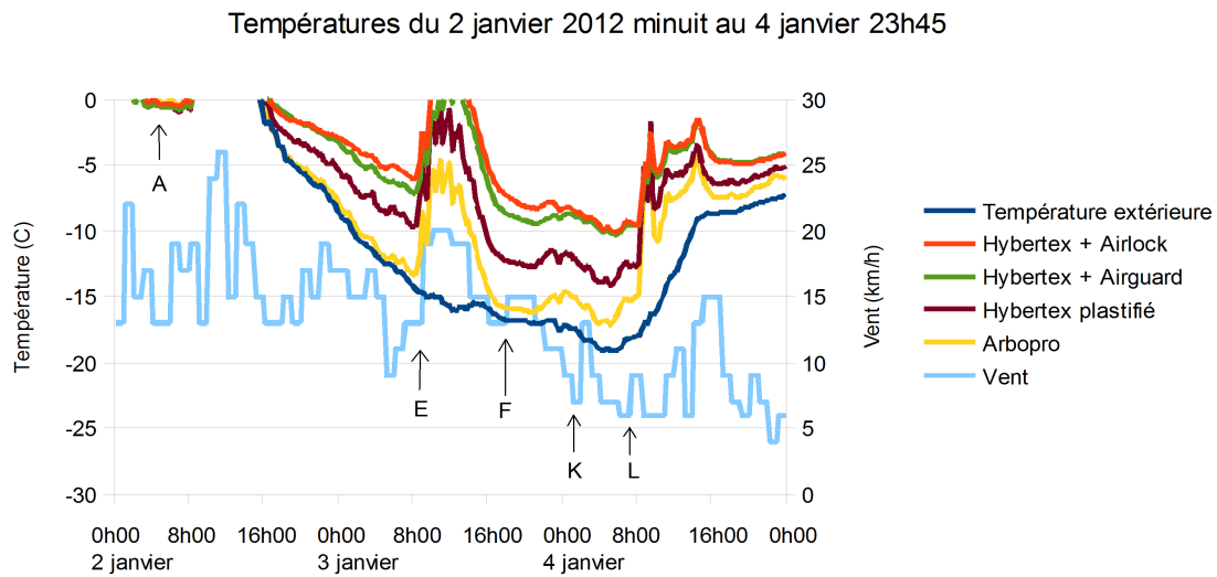
Illustration 10: Températures pour les trois jours du 2 janvier 2012 minuit au 4 janvier 23h45 après une fonte presque totale du couvert nival. Point A = fonte du couvert nival. Point E = lever du soleil et chute de la température extérieure. Point F = coucher du soleil et chute de température. Point K = diminution du vent. Point L = lever du soleil.
