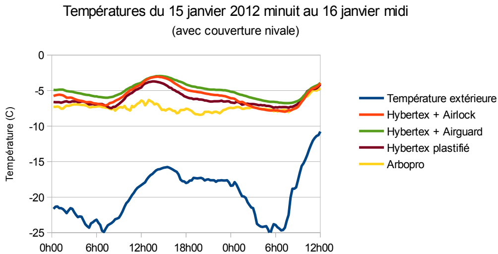
Illustration 9: Nuit la plus froide. Température du 15 janvier 2012 minuit au 16 janvier midi, avec un couvert nival complet.
