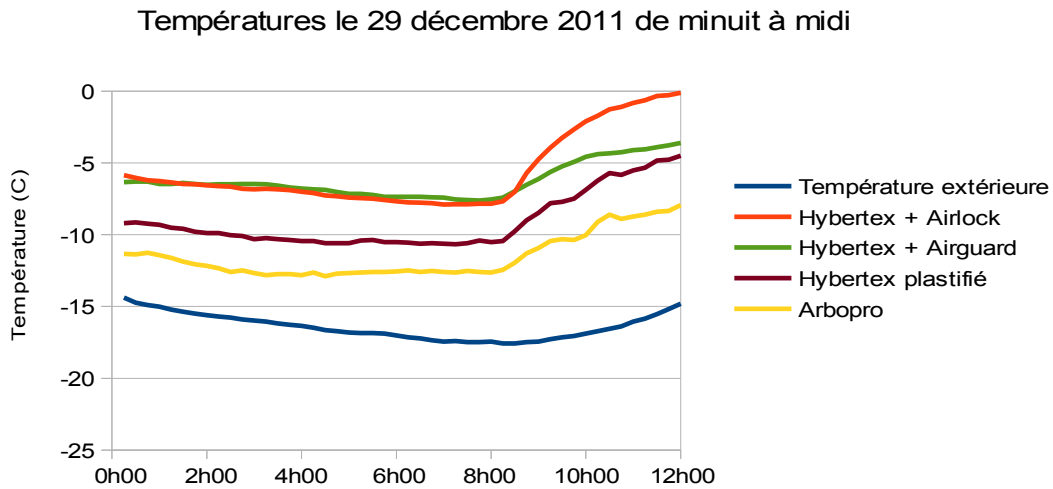
Illustration 8: Températures le 29 décembre 2011 de minuit à midi, froid sans couvert nival.
